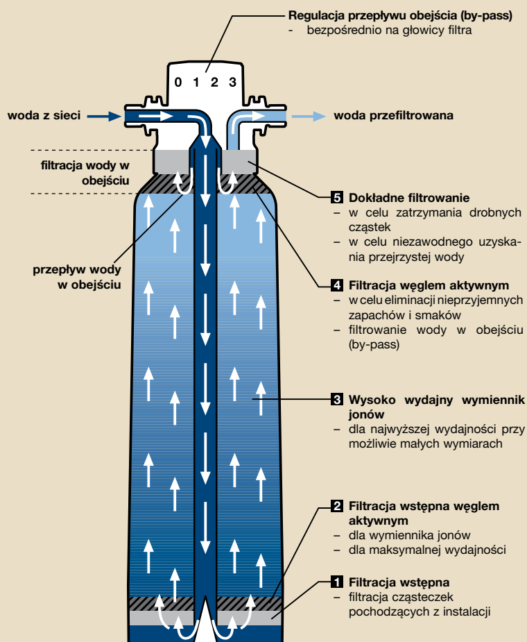
Schemat wkładu filtracyjnego BWT bestmax PREMIUM z 5-stopniową filtracją
